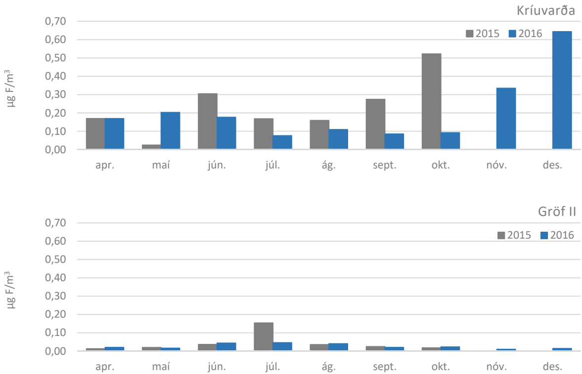
MYND 4.5 Meðalstyrkur heildarflúors í hverjum mánuði á Kríuvörðu og Gröf II árið 2016 og árið 2015 til samanburðar
