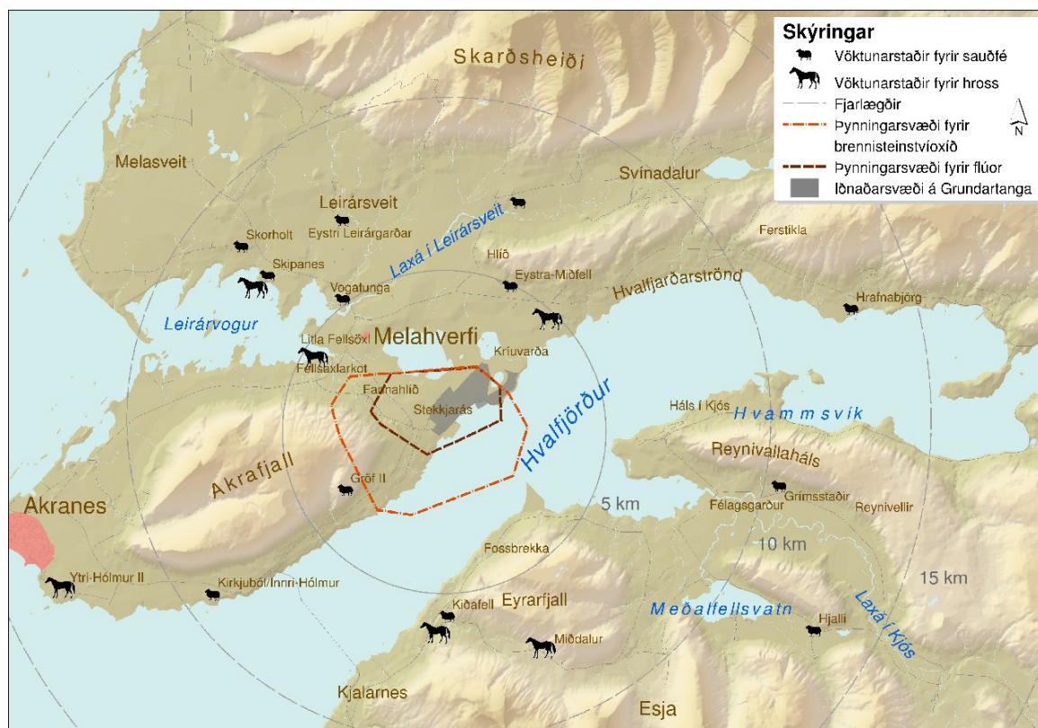
MYND 10.1 Vöktunarsaðir fyrir sauðfé og hross árið 2016
