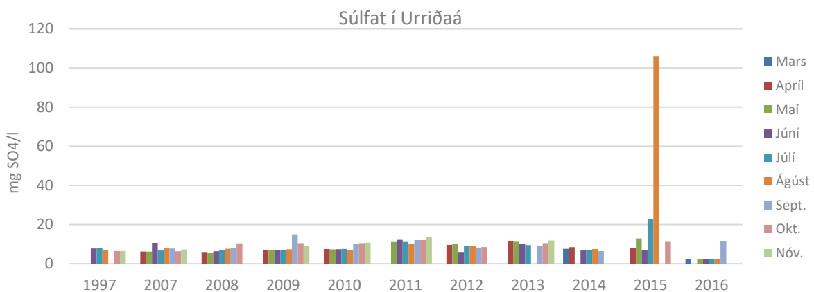
MYND C.4 Meðalstyrkur súlfats í hverjum mánuði í Urriðaa árin 2007 – 2016 og bakgrunnsgildi frá 1997 til viðmiðunar
