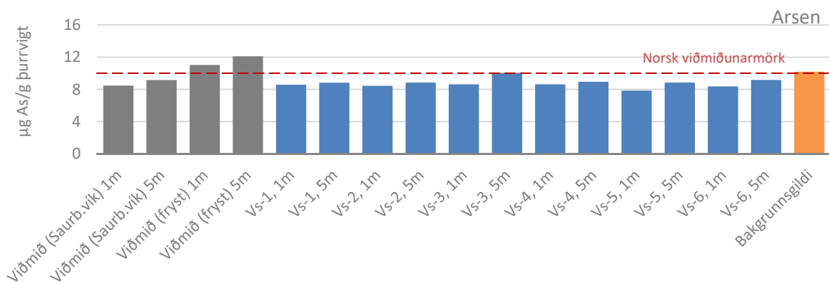
MYND 7.2 Styrkur arsens í mjúkvæf kræklinga 2016, bakgrunnsgildi fyrir styrk arsens í kræklingi frá ómenguðum svæðum við Ísland og norsk viðmiðunarmörk
