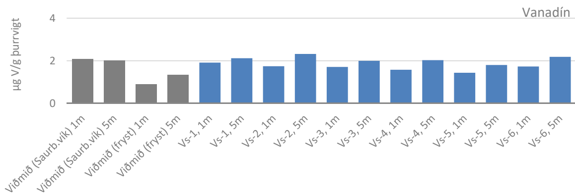
MYND D.4 Styrkur vanadíns í mjúkvæf kræklinga 2016
