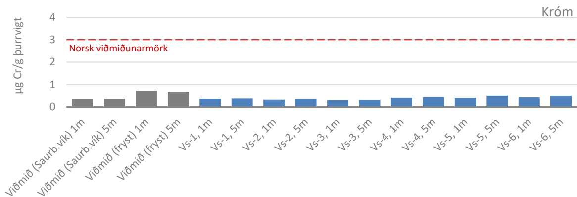
MYND 7.7 Styrkur króms í mjúkvef kræklings 2016 ásamt norskum viðmiðunarmörkum
