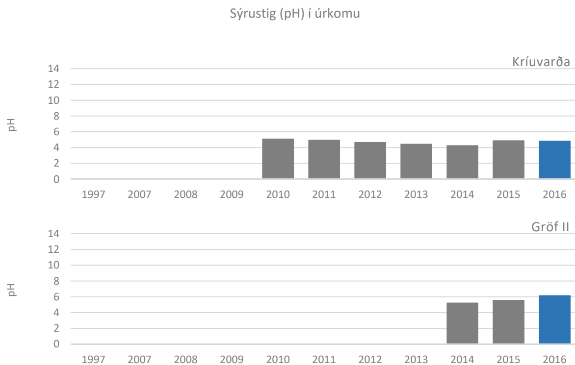
MYND 4.24 Meðal sýrustig í úrkomu á Krúuvörðu og Gröf II
