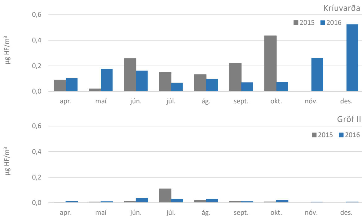
MYND 4.3 Meðalstyrkur loftkennds flúors á Kríuvörðu og Gröf II í hverjum mánuði árið 2016 og til samanburðar árið 2015
