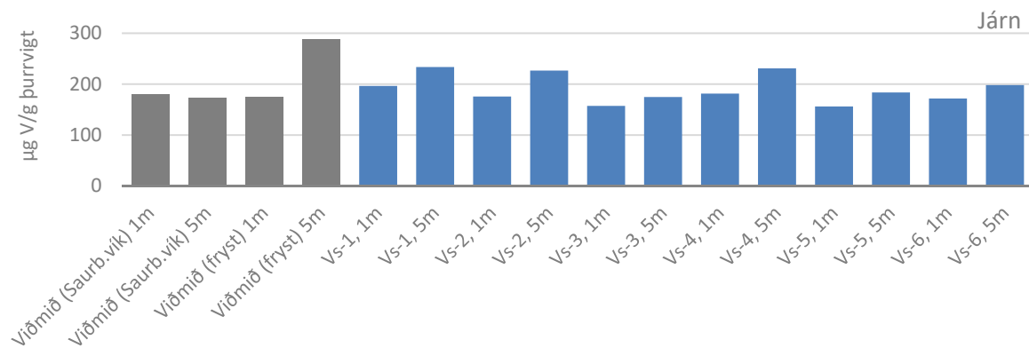
MYND D.3 Styrkur járns í mjúkvæf kræklinga 2016
