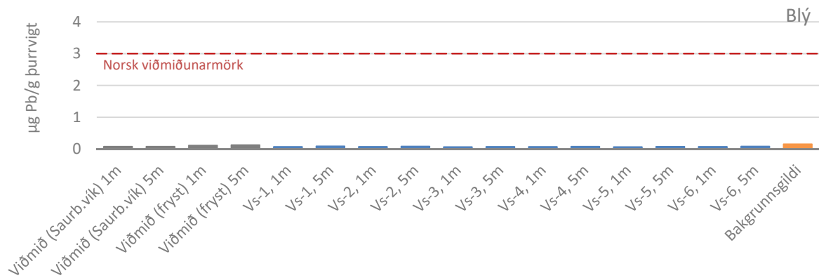
MYND 7.3 Styrkur blýs í mjúkvaf kræklings 2016 ásamt norskum viðmiðunarmörkum
