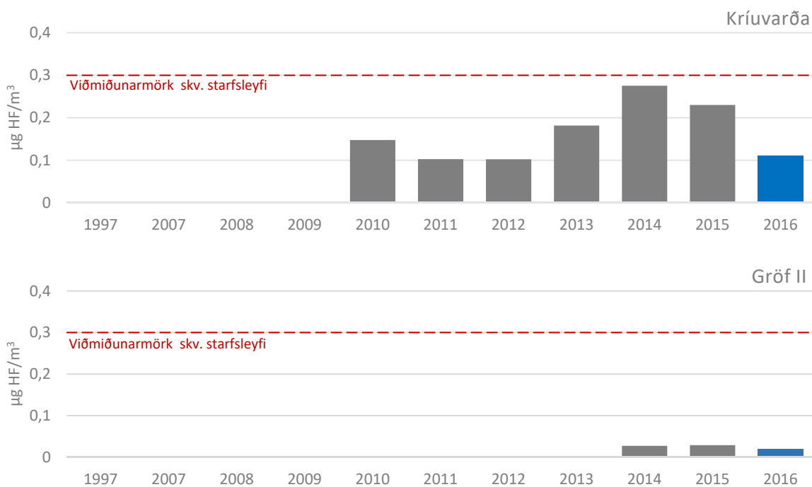
MYND 4.2 Meðalstyrkur loftkennds flúors (HF) í andrúmslofti á vöktunartímabilinu (apríl - október) á Kríuvörðu og Gröf II, ásamt viðmiðunarmörkum samkvæmt starfsleyfi Norðuráls sem gilda utan þýnningarsvæðis
