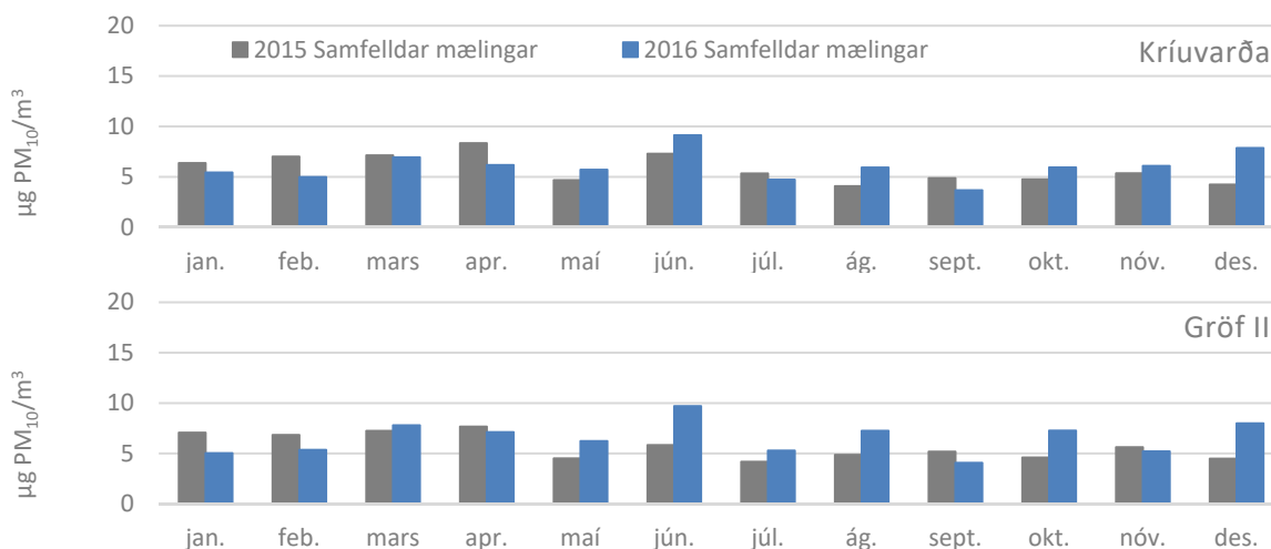
MYND 4.17 Meðalstyrkur svifryks (PM 10 ) í hverjum mánuði á Kríuvörðu og Gröf II árið 2016 og árið 2015 til samanburðar
