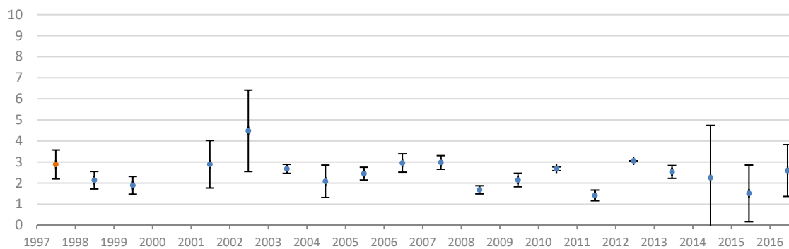
MYND C.12 Meðaltal flúor/kloríðs hlutfalls í Berjadalsá samt 95% öryggisbilum
