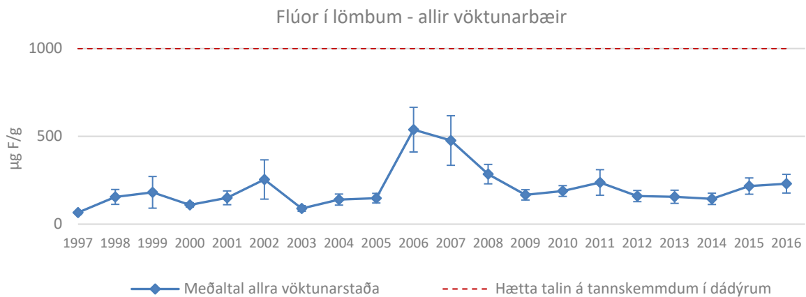
MYND G.1 Meðalstyrkur flúors í lömbum allra vöktunarbæja ásamt 95% öryggisbilum frá 1997 – 2016
