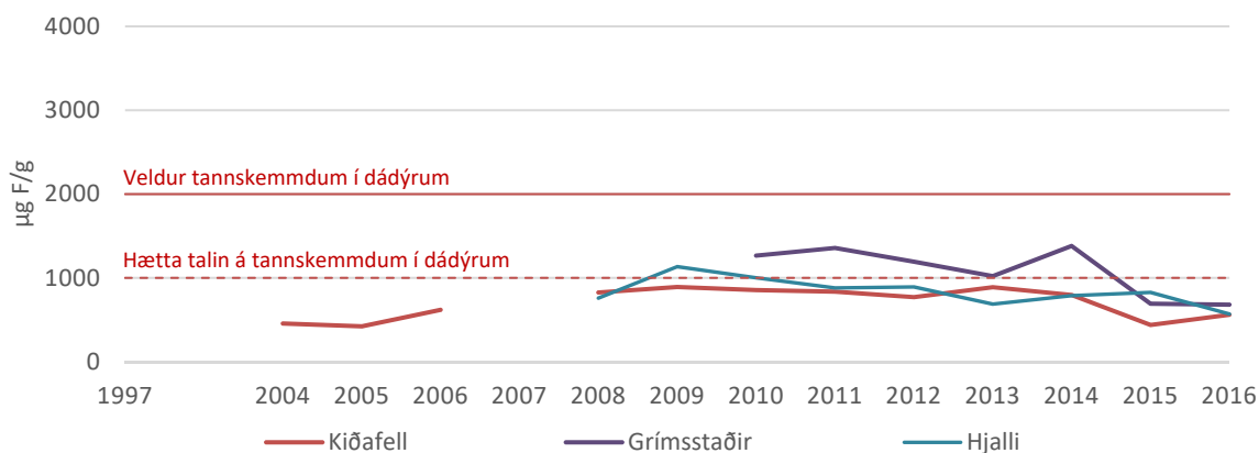
MYND 10.11 Meðalstyrkur flúors í kjálkabeinum fullorðins fjár árin 2007 - 2016 frá bæjum sunnan Hvalfjarðar, og viðmiðunarsýni frá 1997
