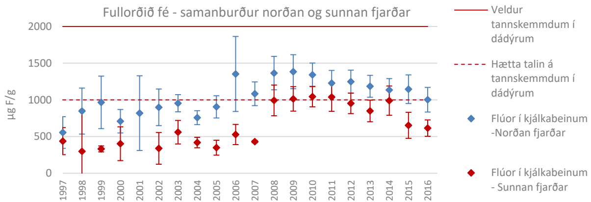
MYND G.8 Samanburður á flúor í beinösku fullorðins fjár norðan og sunnan Hvalfjarðar 1997-2016
