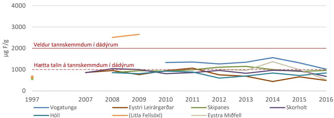
MYND 10.10 Meðalstyrkur flúors í kjálkabeinum fullorðins fjár árin 2007 - 2016 frá bæjum norður og norðvestur af iðnaðarsvæðinu, og viðmiðunarsýni frá 1997
