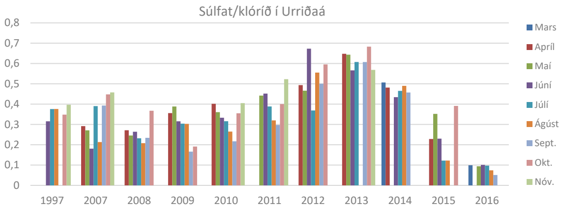
MYND C.3 Hlutfall súlfats/klóríðs í Urriðaa árin 2007 – 2016 og bakgrunnsgildi frá 1997 til viðmiðunar
