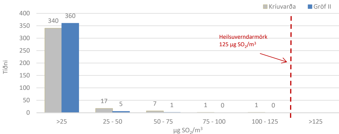
MYND 4.10 Fjöldi mælinga á sólarhringsmeðalstyrk SO 2 á Kríuvörðu og Gröf II, allt árið 2016
