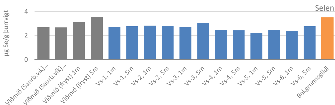
MYND D.1 Styrkur selens í mjúkvef kræklinga 2016
