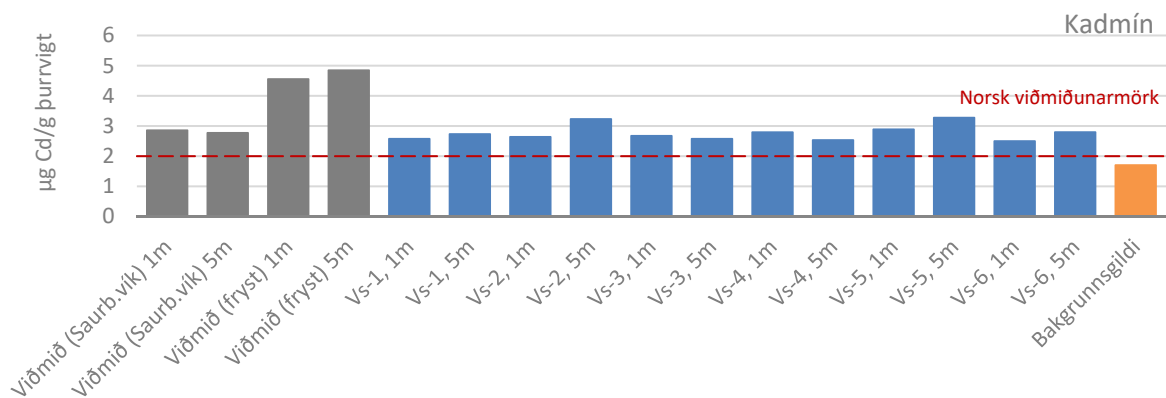
MYND 7.5 Styrkur kadmíns í mjúkvæf kræklinga 2016, bakgrunnsgildi fyrir styrk kadmíns í kræklingi frá ómengduðum svæðum við Ísland og norsk viðmiðunarmörk
