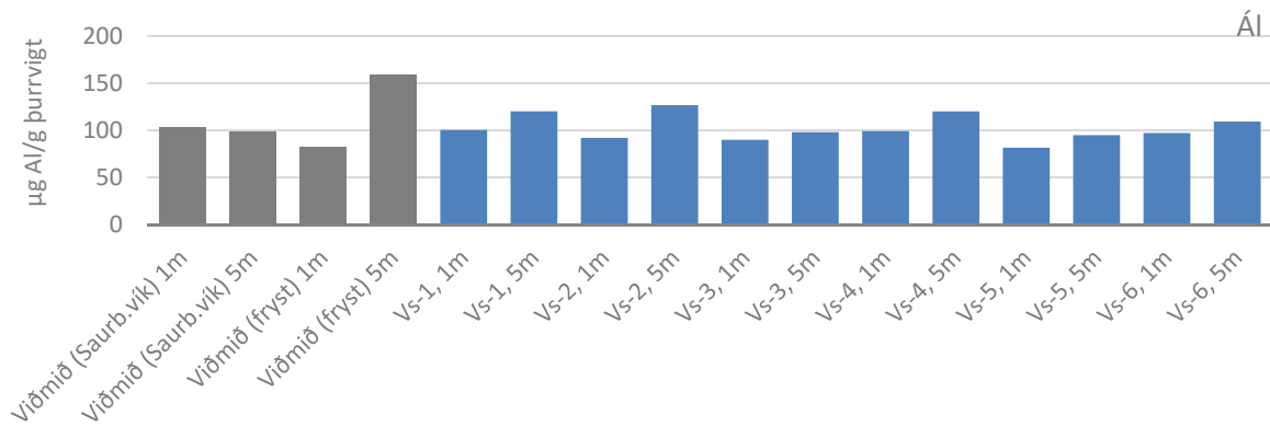
MYND D.2 Styrkur áls í mjúkvæf kræklinga 2016
