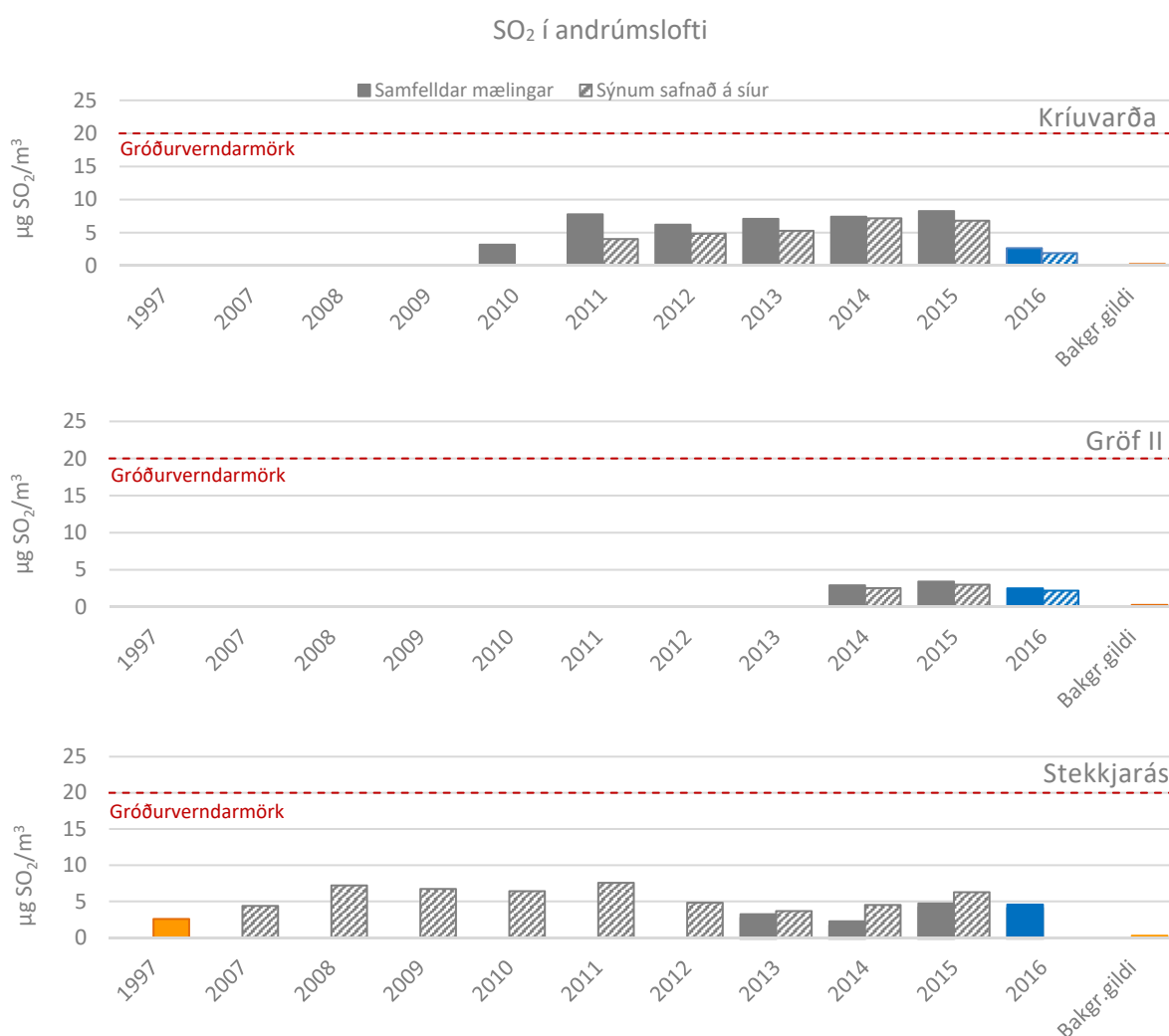
MYND 4.7 Meðalstyrkur \text{SO}_2 á vöktunartímabilinu (apríl - október) á Kríuvörðu, Gröf II og Stekkjarási ásamt gróðurverndarmörkum. Bakgrunnsgildi mæld við Írafoss árið 2003 ( 0,26 \mu\text{g SO}_2/\text{m}^3 )
