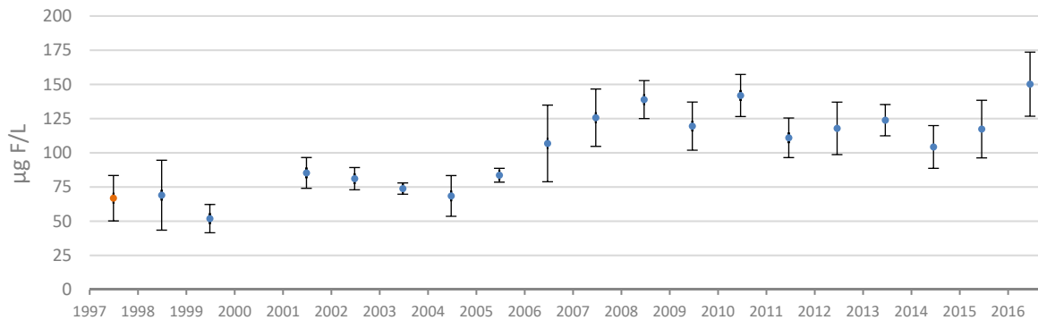
MYND C.11 Meðalstyrkur flúors í Urriðá á samt 95% öryggisbilum
