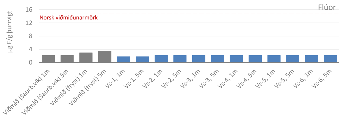
MYND 7.4 Styrkur flúors í mjúkvaf kræklings 2016 ásamt norskum viðmiðunarmörkum
