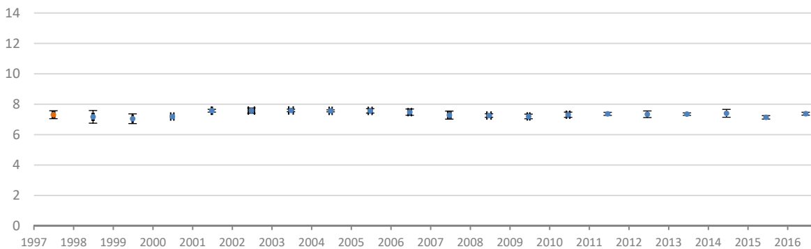
MYND C.6 Meðaltal sýrustigs í Urriðaá mælt 1997 – 2016 ásamt 95% öryggisbilum
