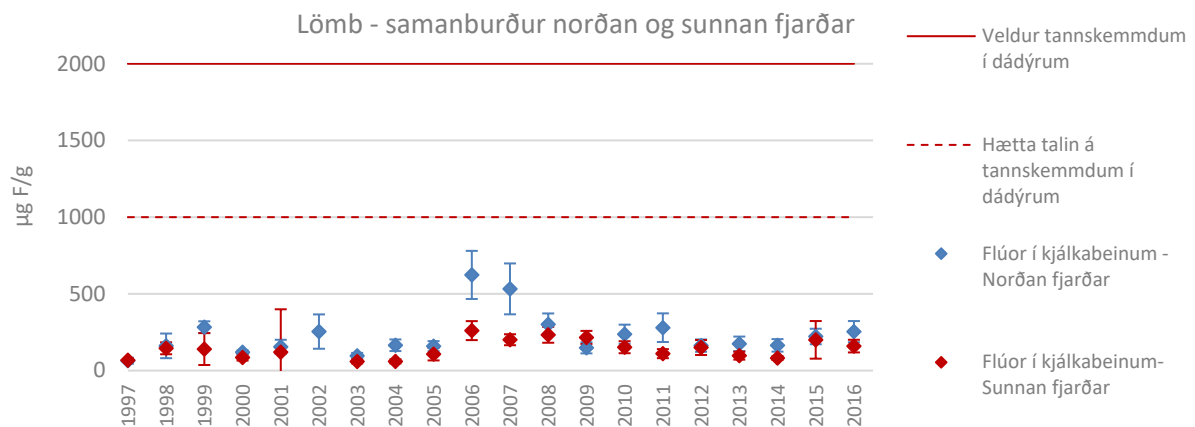
MYND G.2 Samanburður á meðalstyrk flúors í beinösku lamba, norðan og sunnan Hvalfjarðar 1997-2016
