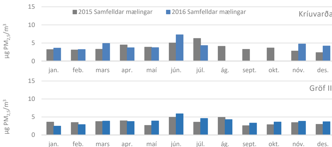
MYND 4.18 Meðalstyrkur svifryks (PM 2,5 ) í hverjum mánuði á Kríuvörðu og Gröf II árið 2016 og árið 2015 til samanburðar
