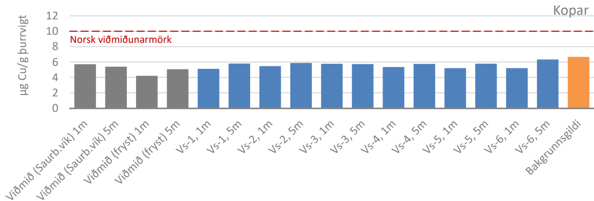
MYND 7.6 Styrkur kopars í mjúkvef kræklings 2016, bakgrunnsgildi fyrir styrk kopars í kræklingi frá ómenguðum svæðum við Ísland og norsk viðmiðunarmörk
