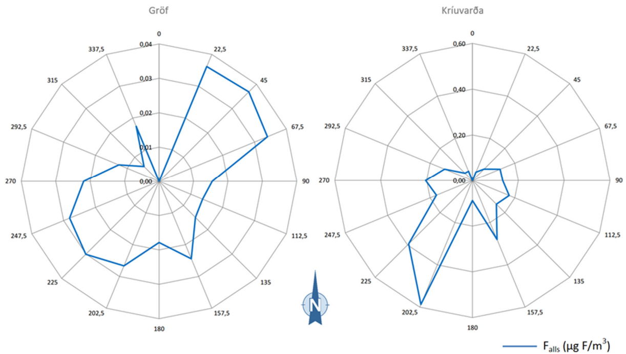
MYND 4.6 Styrkur flúors ( \mu\text{g F/m}^3 ) eftir vindáttum frá apríl – október 2016 á Kríuvörðu og Gröf II. Gröfin eru ekki í sama kvarða
