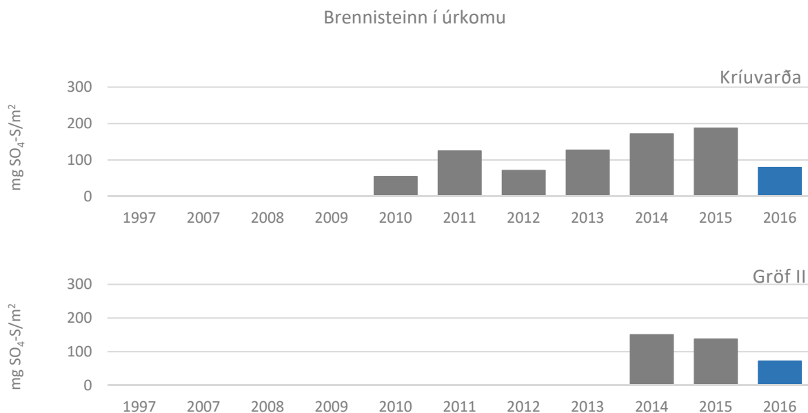
MYND 4.23 Áfallsgildi brennisteins í úrkomu á Krúuvörðu og Gröf II á vöktunartímabilinu (apríl – október) árið 2016
