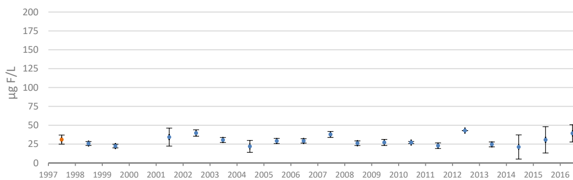
MYND C.13 Meðalstyrkur flúors í Berjadalsá samt 95% öryggisbilum
