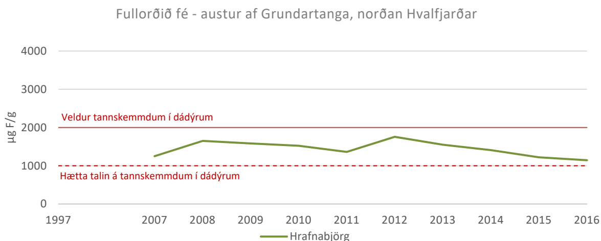
MYND 10.8 Meðalstyrkur flúors í kjálkabeinum fullorðins fjár árin 2007 - 2016 frá bæjum austur af iðnaðarsvæðinu, og viðmiðunarsýni frá 1997
