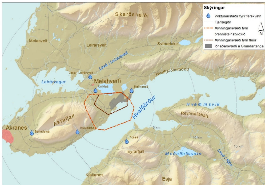
MYND 5.1 Vöktunarstaðir fyrir ferskvatn í Hvalfirði árið 2016
