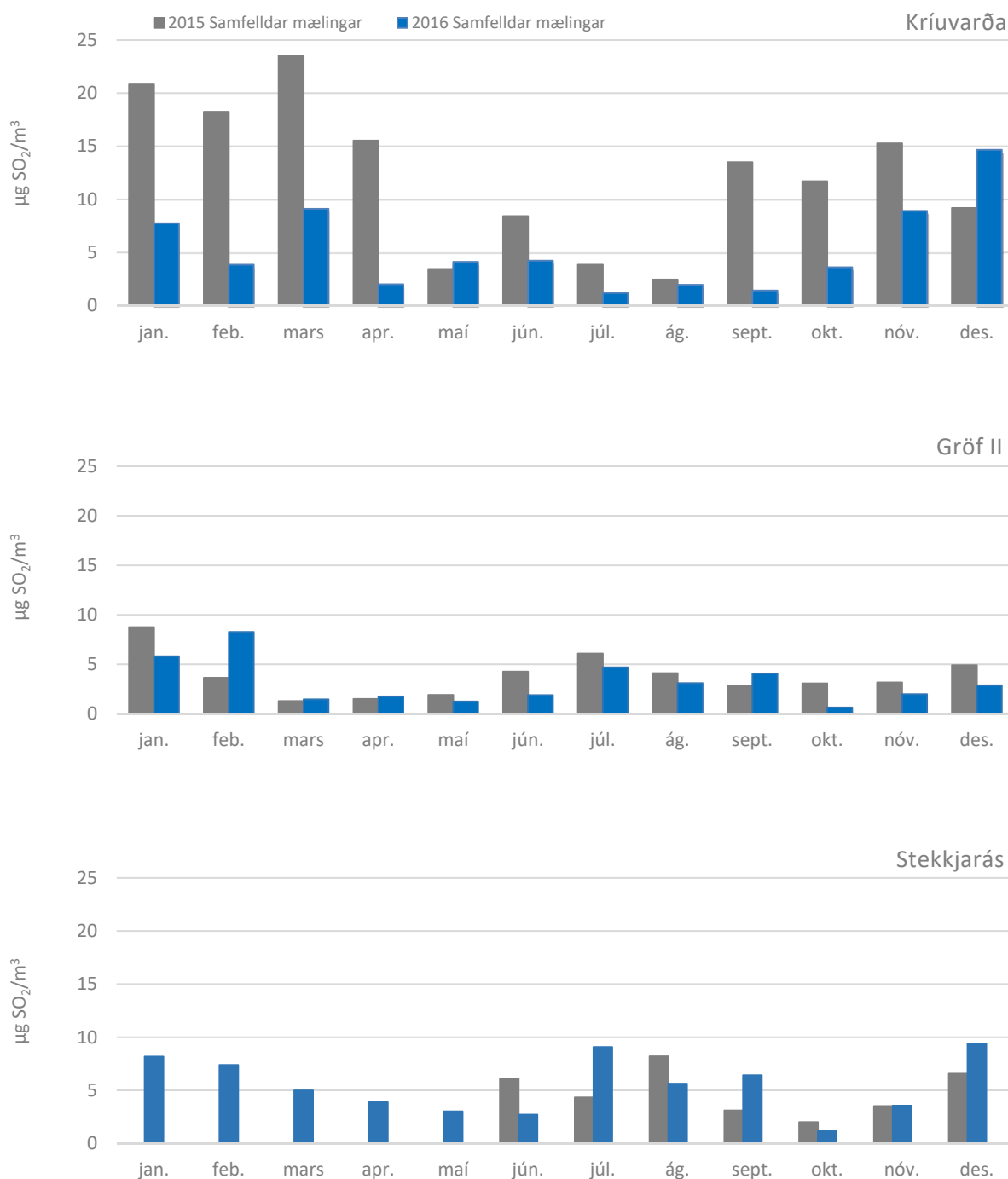
MYND 4.9 Meðalstyrkur brennisteinstvíoxíðs í andrúmslofti í hverjum mánuði á Krúvörðu, Gröf II og Stekkjarási árið 2016 og árið 2015 til samanburðar
