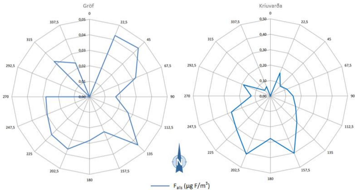
MYND 4.4 Styrkur flúors (µg F/m 3 ) eftir vindáttum árið 2017 á Kríuvarða og Gröf II. Gröfin eru ekki í sama kvarða.
