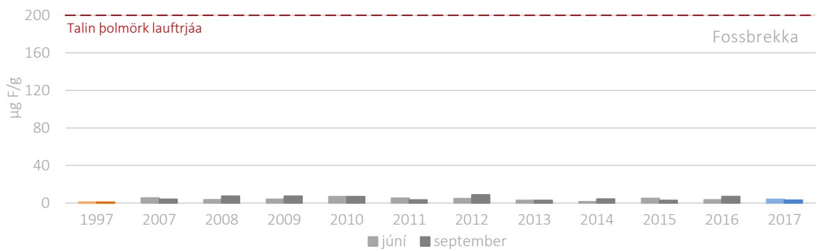
MYND F.2 (framhald) Meðalstyrkur flúors í laufi, vor og haust árin 2007 – 2017 og bakgrunnsgildi frá 1997 til viðmiðunar.
