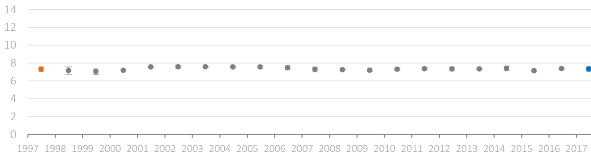
MYND C.4 Meðaltal sýrustigs í Urriðá mælt 1997 – 2017 ásamt 95% öryggisbilum.
