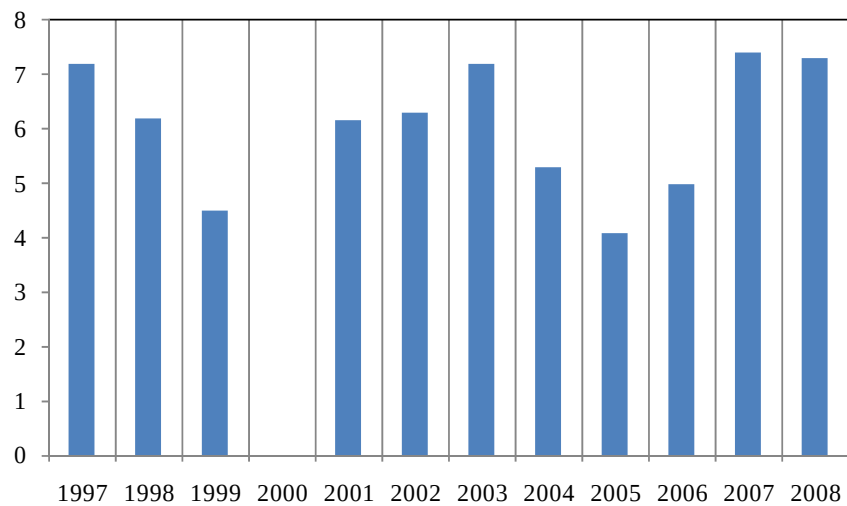
Mynd 7.9 Ársmeðaltal súlfats í Urriðaa 1997-2008 (bakgrunns­mælingar frá 1997). Mælingar fóru ekki fram árið 2000.
