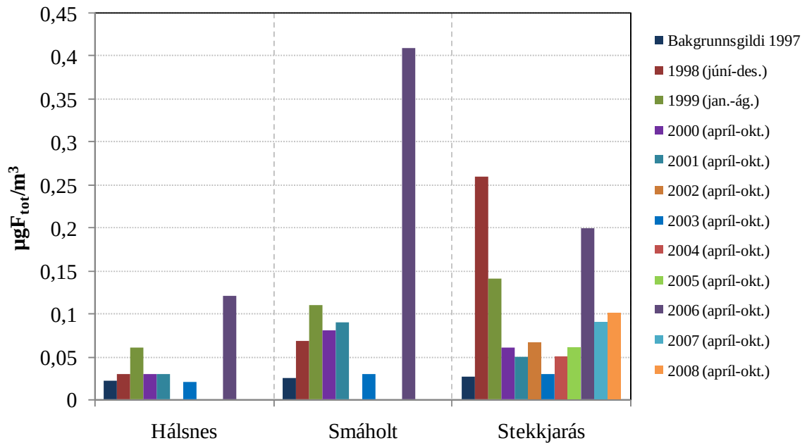
Mynd 4.3 Ársmeðaltöl heildarflúors (F tot ) á vöktunarstöðum árin 1997-2008. Bakgrunnsgildi eru frá árinu 1997. Bilun varð í reykhreinsivirki 1 hjá Norðuráli 24. ágúst 2006. Stekkjarás er innan þýnningarsvæðis.
