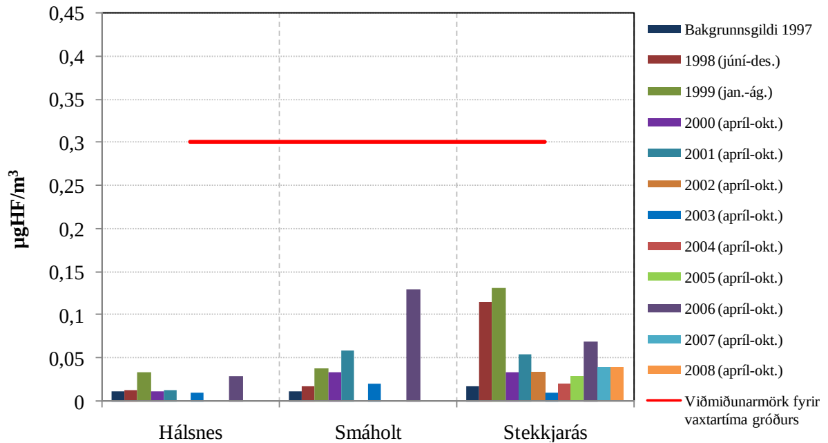
Mynd 4.2 Ársmeðaltöl HF á vöktunarstöðum árin 1997-2008. Bakgrunnsgildi eru frá árinu 1997. Viðmiðunarmörk HF yfir vaxtartíma gróðurs utan þýnningarsvæðis eru sýnd með rauðri línu. Bilun varð í reykhreinsivirki 1 hjá Norðuráli 24. ágúst 2006. Stekkjarás er innan þýnningarsvæðis.
