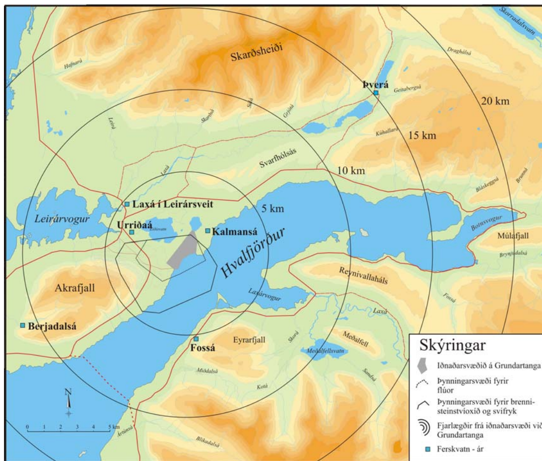
Mynd 7.1 Vöktunarstaðir fyrir ferskvatn í Hvalfirði árið 2008. Ferskvatnssýnum var safnað einu sinni til tvisvar í mánuði frá apríl til október.
