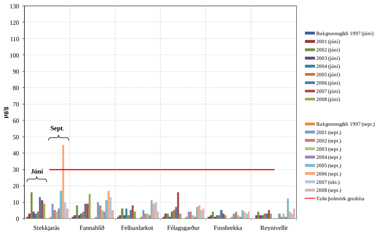
Mynd 5.2 Meðaltal flúors í grasi (samanlagt í þurrefni og skoli) vor og haust 1997-2008 (bakgrunnsgildi er frá 1997). Rauð lína sýnir skilgreind eða talin þolmörk fyrir sauðfé. Bilun varð í reykahreinsivirki 1 hjá Norðuráli 24. ágúst 2006. Stekkjarás er innan þynningarsvæðis fyrir flúor.
