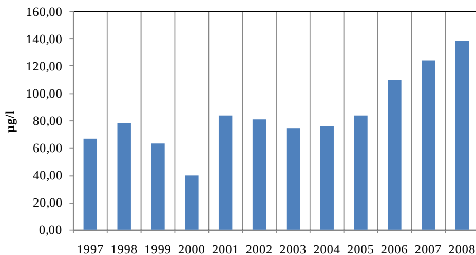
Mynd 7.5 Ársmeðaltal flúoríðs í Urriðaá 1997-2008 (bakgrunnsmælingar frá 1997). Mælingar fóru ekki fram árið 2000.
