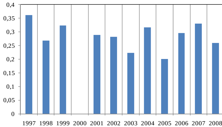
Mynd 7.8 Súlfat/klóríð hlutfall í Urriðaa, ársmeðaltal 1997-2008 (bakgrunns­mælingar frá 1997). Mælingar fóru ekki fram árið 2000.
