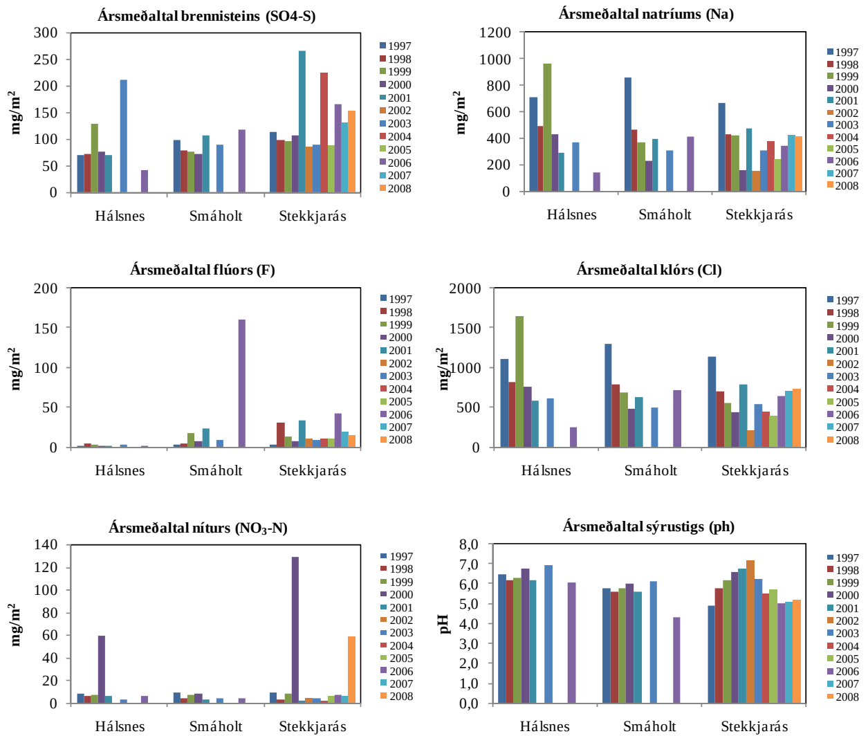
Mynd 4.10 Ársmeðaltöl ýmissa efna og sýrustigs í úrkomu árin 1997-2008. Bakgrunnsmælingar eru frá 1997. Stekkjarás er innan þýnningarsvæðis.
