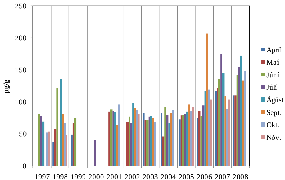
Mynd 7.3 Flúoríð styrkur í Urriðaá fyrir hvern mælímánuð árin 1997-2008 (bakgrunnsmaðlingar frá 1997). Mælingar fóru ekki fram árið 2000.
